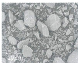
高清掃シリカSEM像(×3000)
