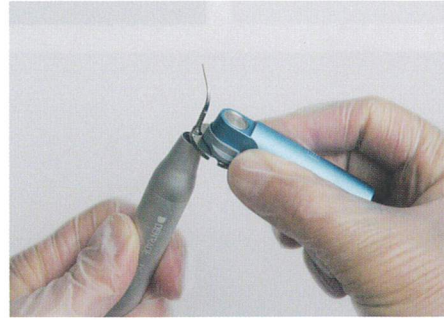
取り外し チップの交換用に専用レンチが付属。チップやハンドピースを傷めることなく交換出来ます。
